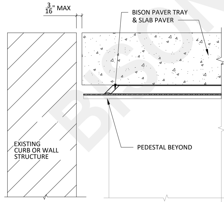
D5 PAVER EDGE AT THRESHOLD OR INTERIOR CURB SCALE: 6" = 1'-0"
