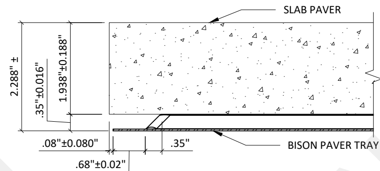
D1 BISON PAVER TRAY/SLAB PAVER WIND SYSTEM EDGE DETAIL SCALE: 6" = 1'-0"
